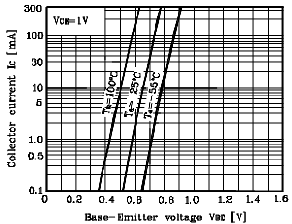
Fig. 2 I_C - V_{BE}
